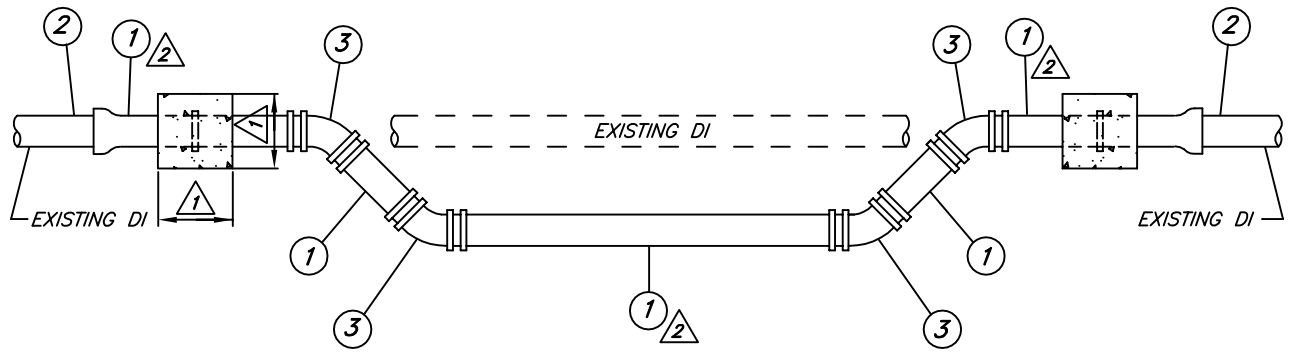
ELEVATION
