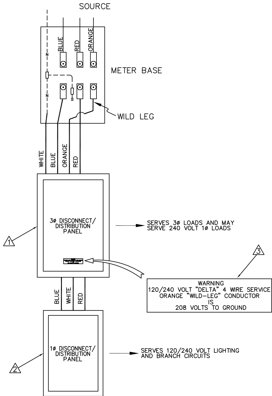
COMBINATION (WILD-LEG) SERVICE 1 \phi /3 \phi - 120/240 VOLT 4 WIRE
